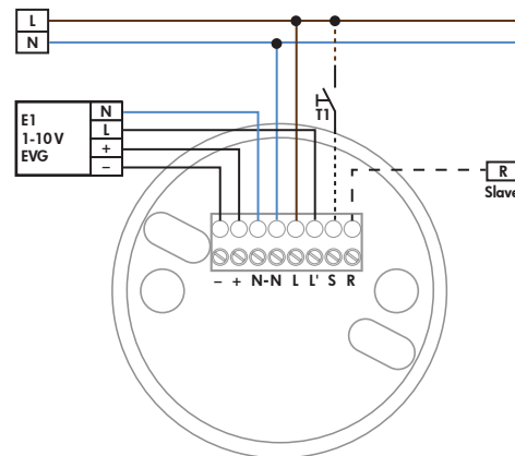
PD4-M-DIM-AP Sockel
