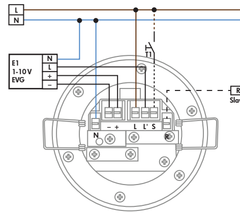
PD4-M-DIM-DE/-UP
